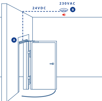
A GEZE EFS VRIJLOOPDRANGER (24V)
